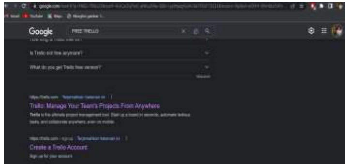
Gambar 1. Mencari Trello
