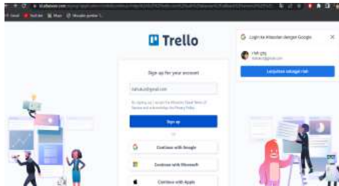
Gambar 2. Verifikasi Email
